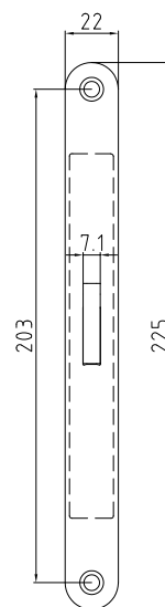
Måttitning, Connect 411-50/70
