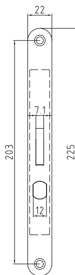
Måttitning, Connect 410-50/70
